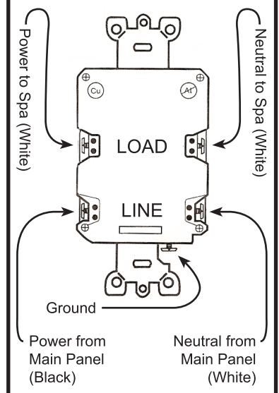
120V GFCI
